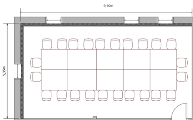
Bestuhlungsbeispiel Blockform
